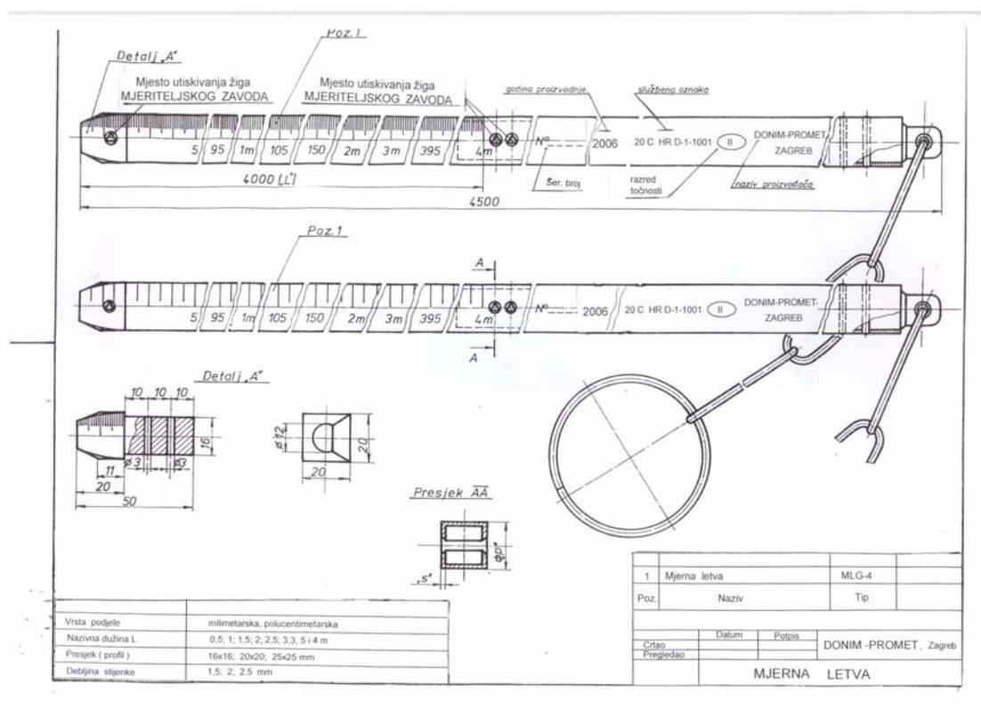
Slika 1: Crtež mjerne letve tipa MLG
